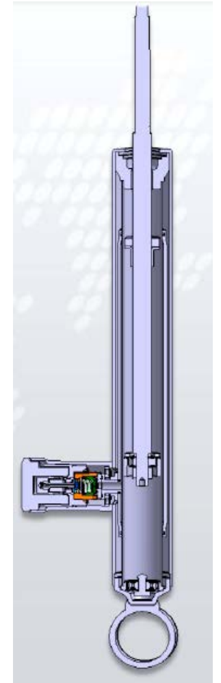
Электронные амортизаторы 3D Design CDC
