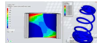
CAE анализ
