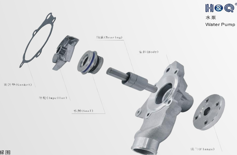
分解图 Exploded view
